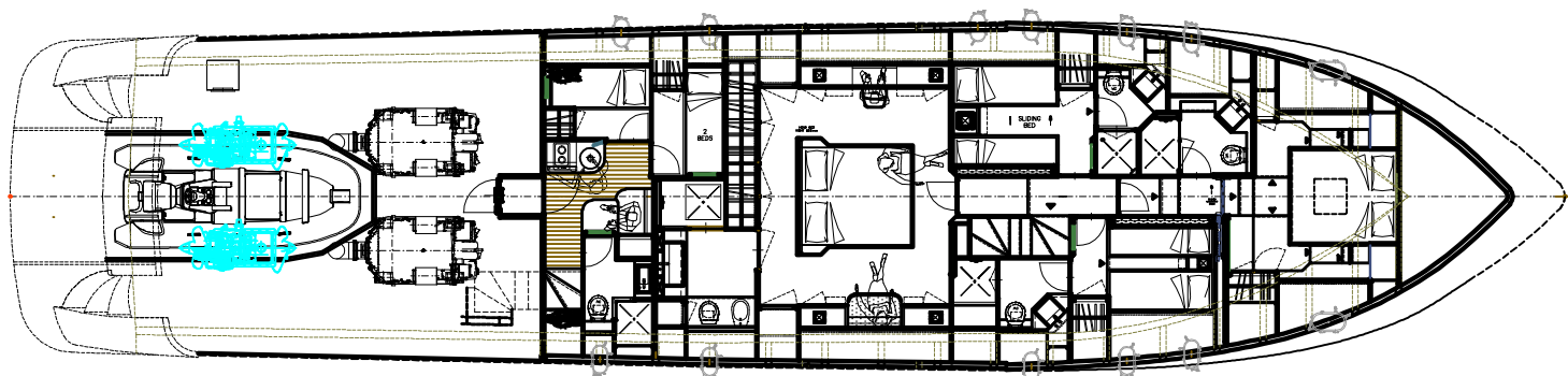
PIANTA PONTE SOTTOCOPERTA
